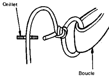
Fig. 4.3 - Schéma de début de laçage
