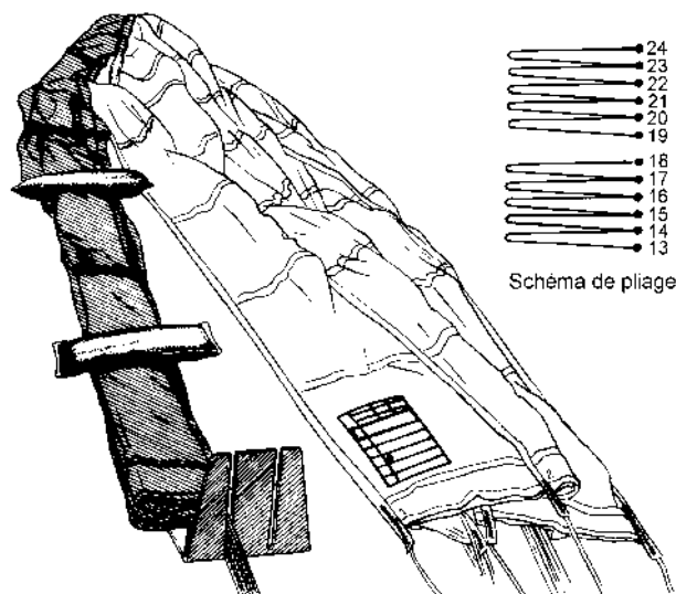
Fig. 4.26 - Insertion des suspentes n°13 à 24
