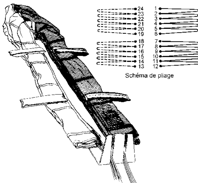
Fig. 4.27 - Insertion des suspentes n°12 à 1
