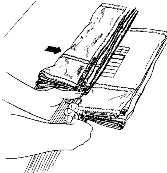
Fig. 4.28 - Superposition des deux parties de voile
