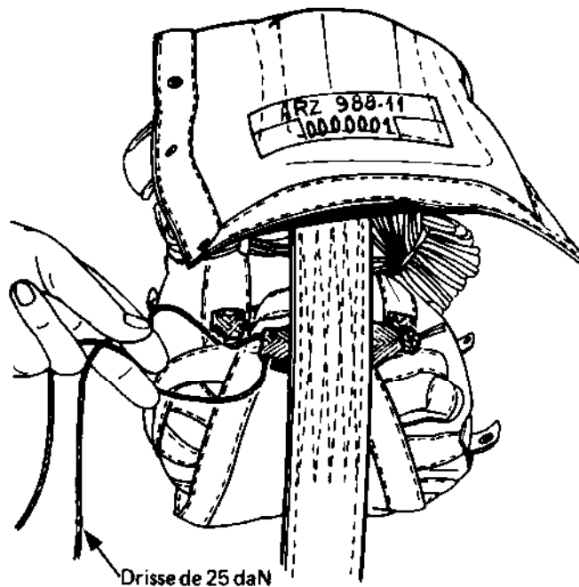
Fig. 4.38 - Mise en place du rabat
