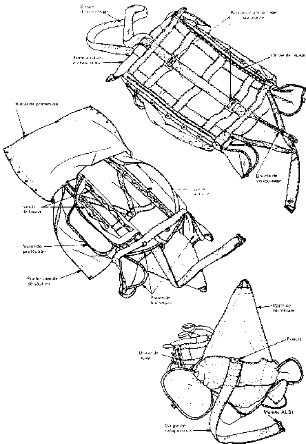
Fig. 2.2 - Sac de voile équipé
